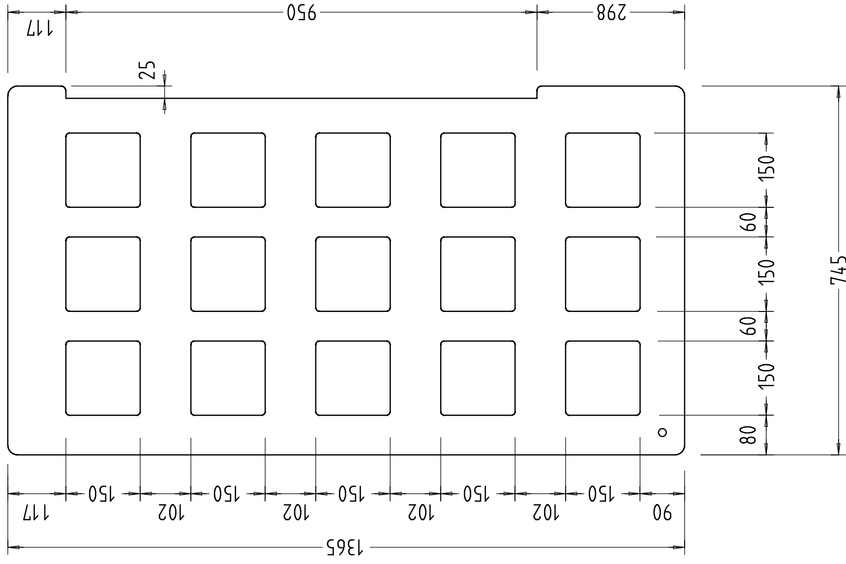
Matratzenauflagerplatte
